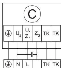
Схема №1 (1-230 В)
