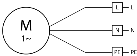
Схема № 1 для однофазных вентиляторов
