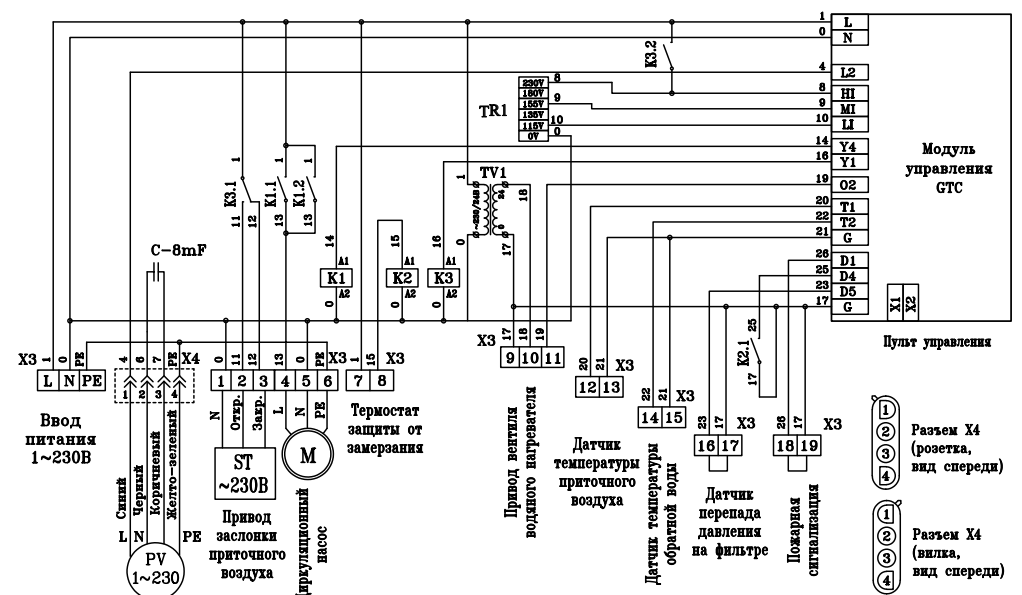
Схема для установок с водяным нагревателем
