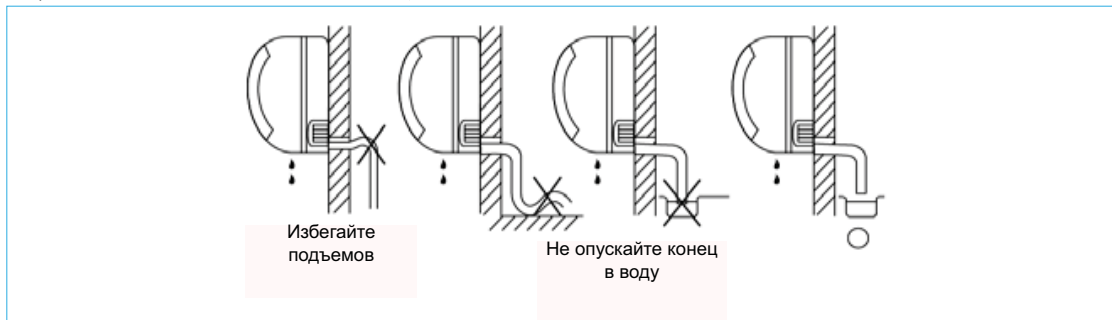
Рисунок №50 Способ прокладки дренажного трубопровода
